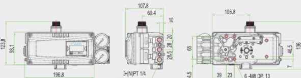
YT-3301 本体
